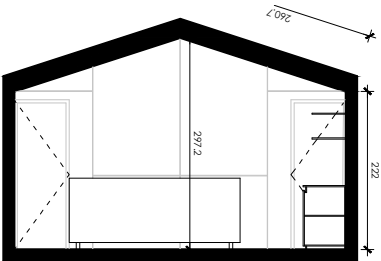
CORTE LATERAL
